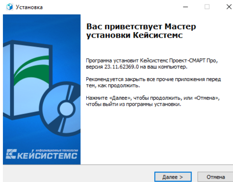
Рисунок 34. Мастер установки
