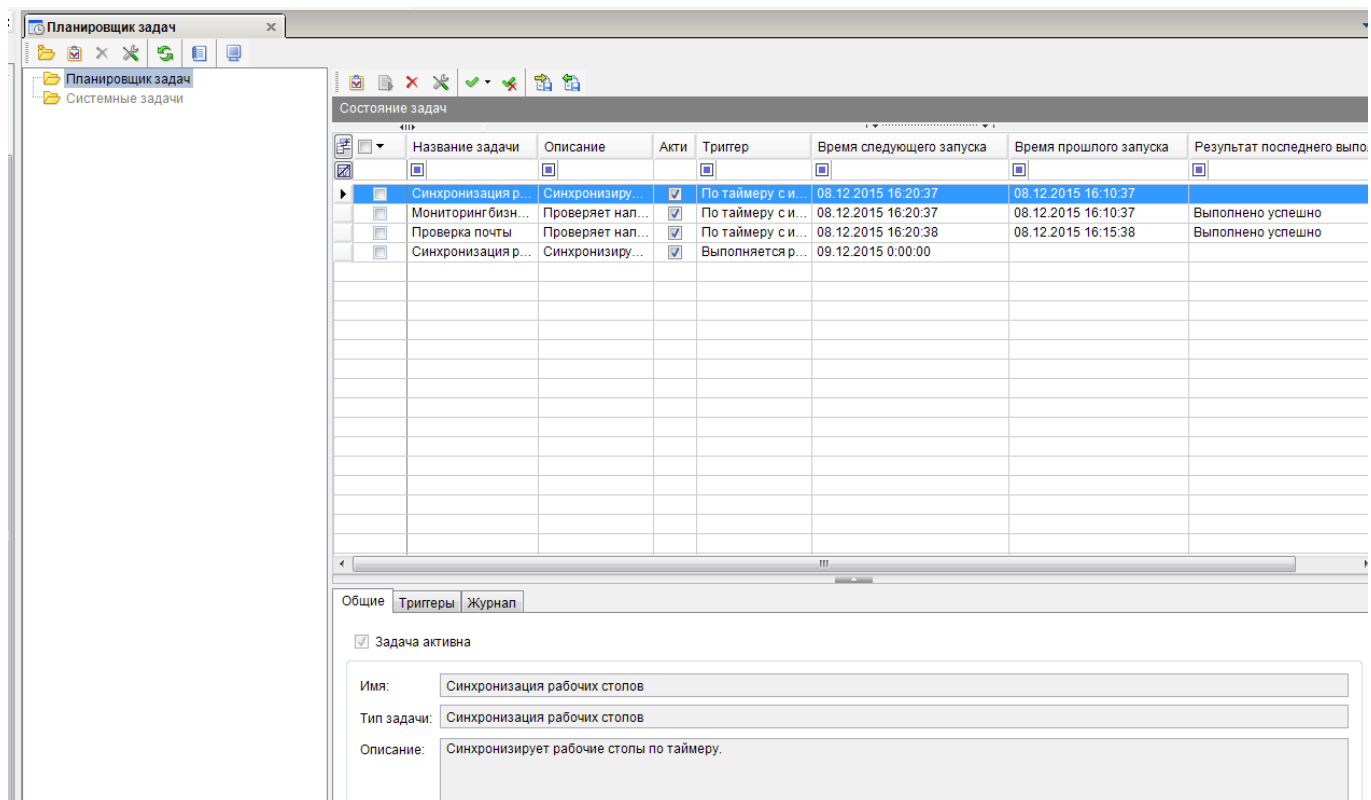
Рисунок 48. Планировщик задач
