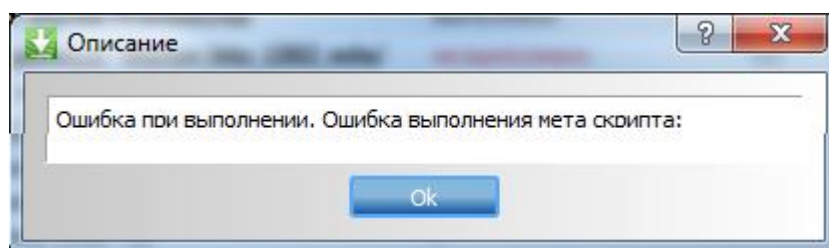
Рисунок 18. Пример ошибки
