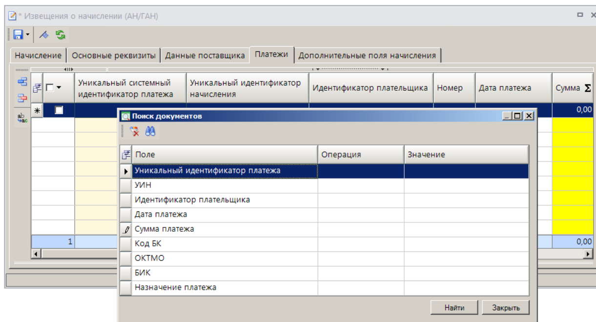
Рисунок 42. Окно поиска платежей для квитирования
