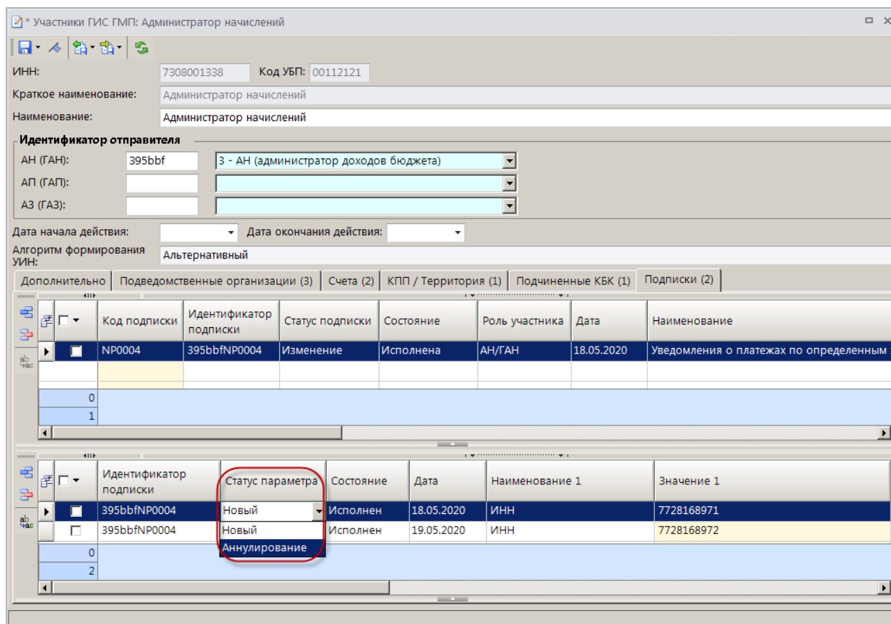
Рисунок 92. Окно редактирования данных участника ГИС ГМП, удаление параметров подписки
