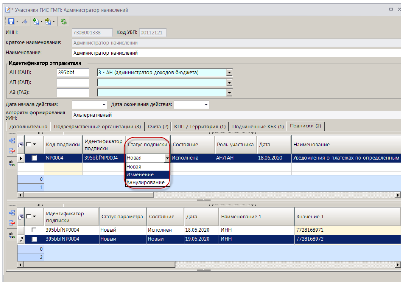
Рисунок 89. Окно редактирования данных участника ГИС ГМП, добавление параметров подписки
