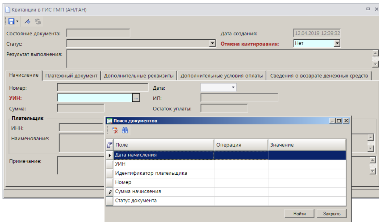
Рисунок 44. Окно ввода/редактирования квитанции, вкладка Начисление
