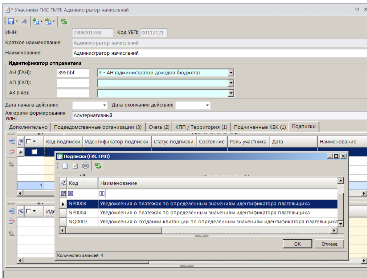
Рисунок 81. Окно выбора подписок
