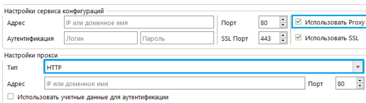
Рисунок 9. Настройка прокси
