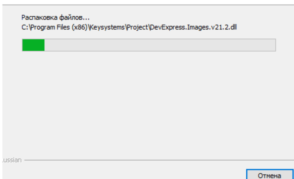
Рисунок 34. Процесс установки
