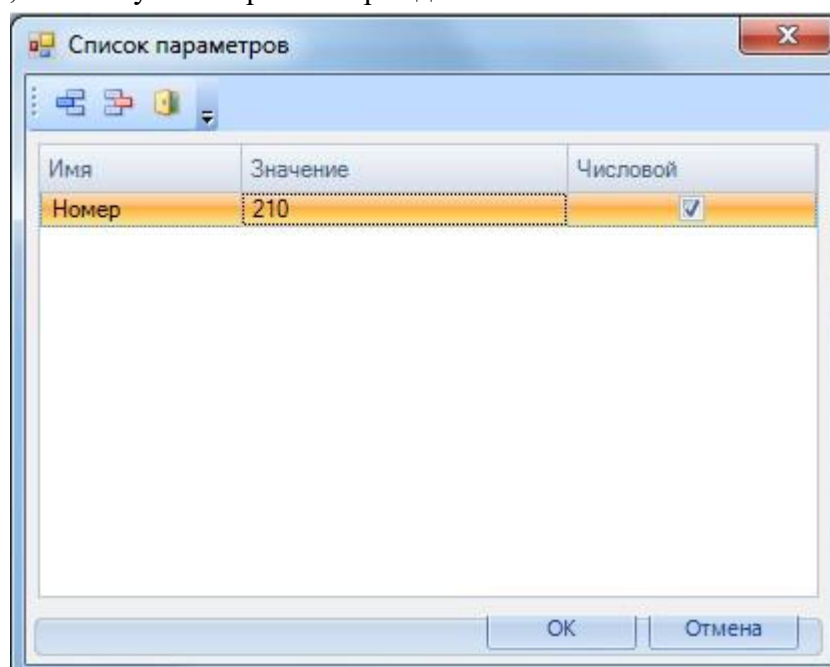
Рисунок 65. Список параметров
