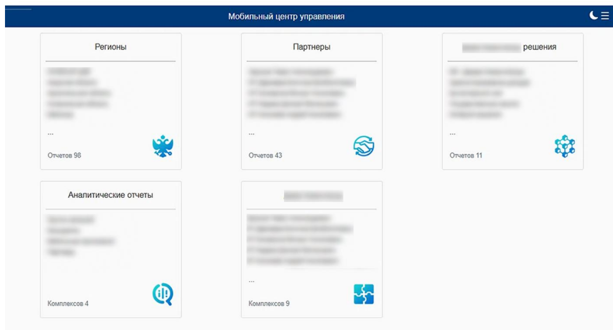
Рисунок 2. Главный экран
