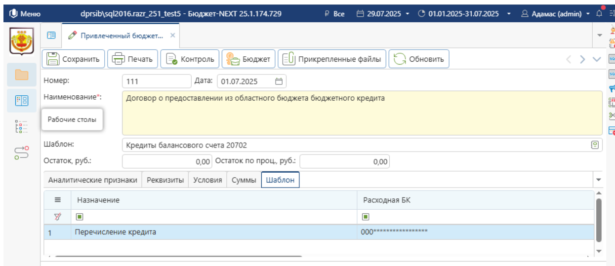
Рисунок 5 Аналитические признаки
