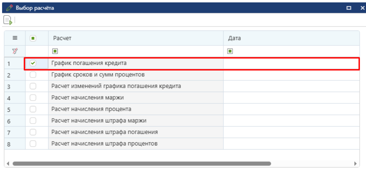
Рисунок 15 Выбор расчета
