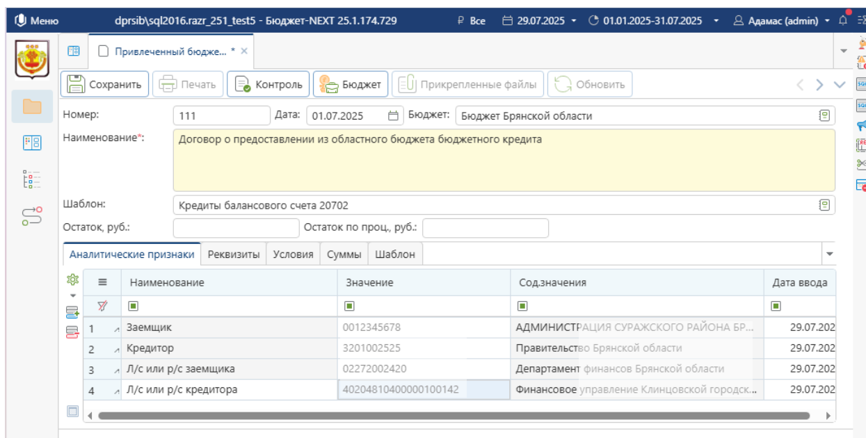
Рисунок 4 Вкладка «Шаблон»
