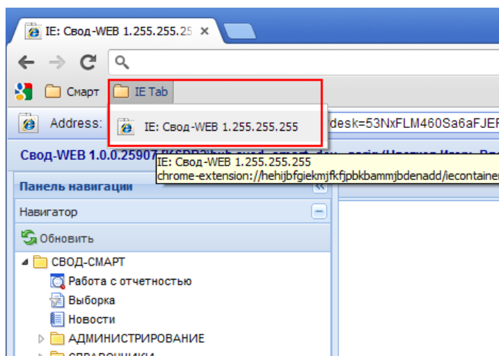
Рисунок 8. Запуск Свод-web
