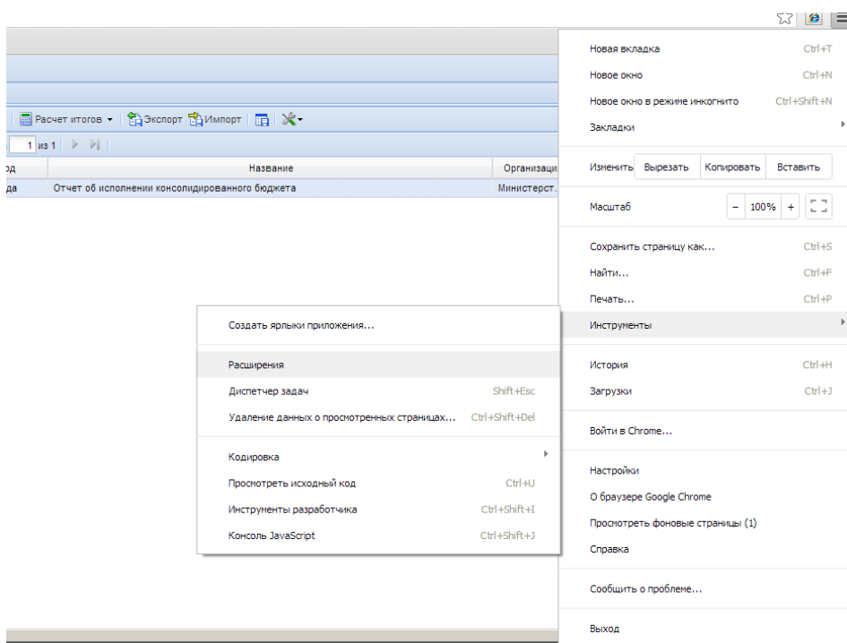
Рисунок 1. Расширения
