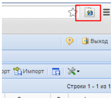
Рисунок 5. Страница «Свод-веб»
