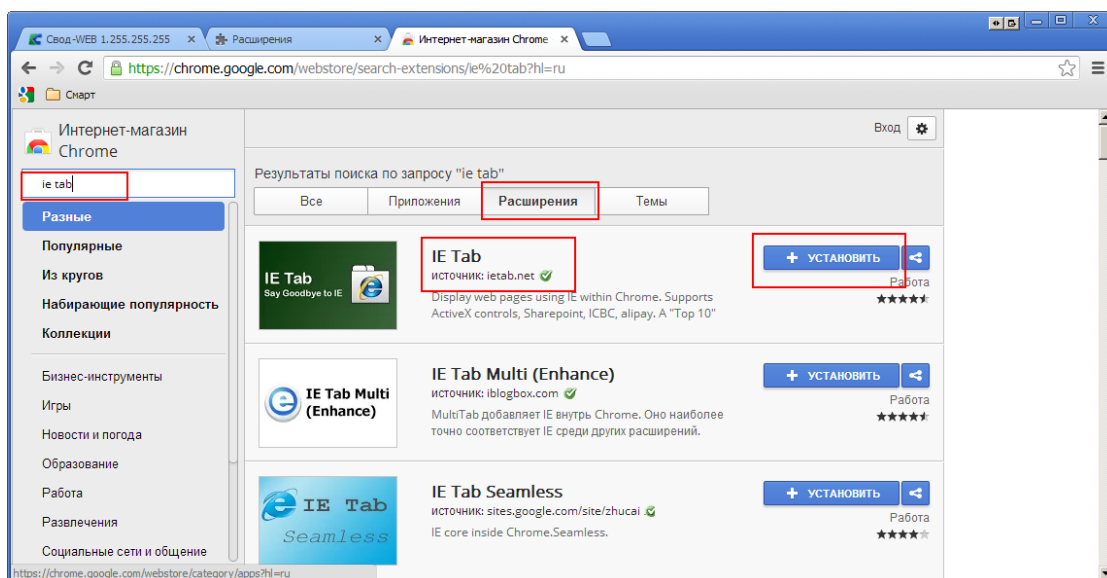
Рисунок 3. Список расширений
