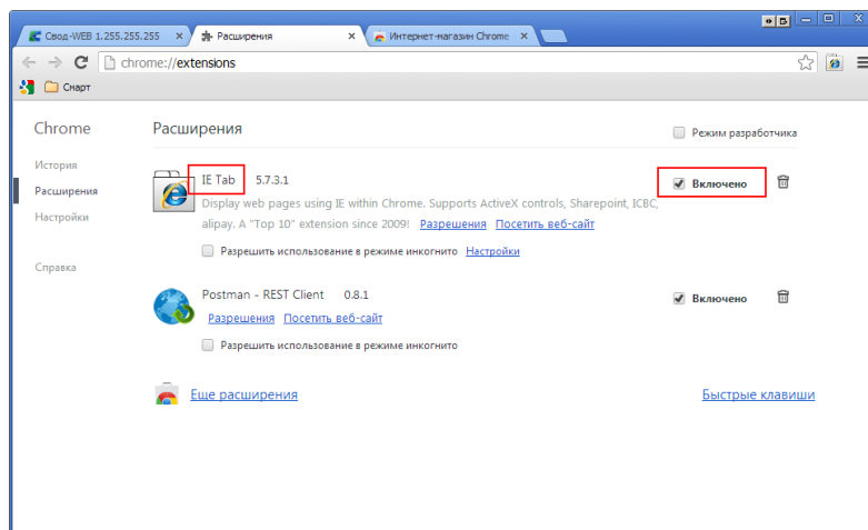
Рисунок 2. Настройка расширения
